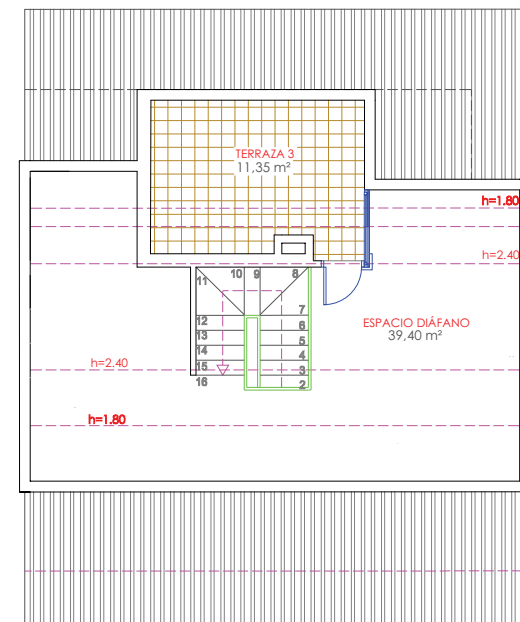
PLANTA BAJO CUBIERTA
