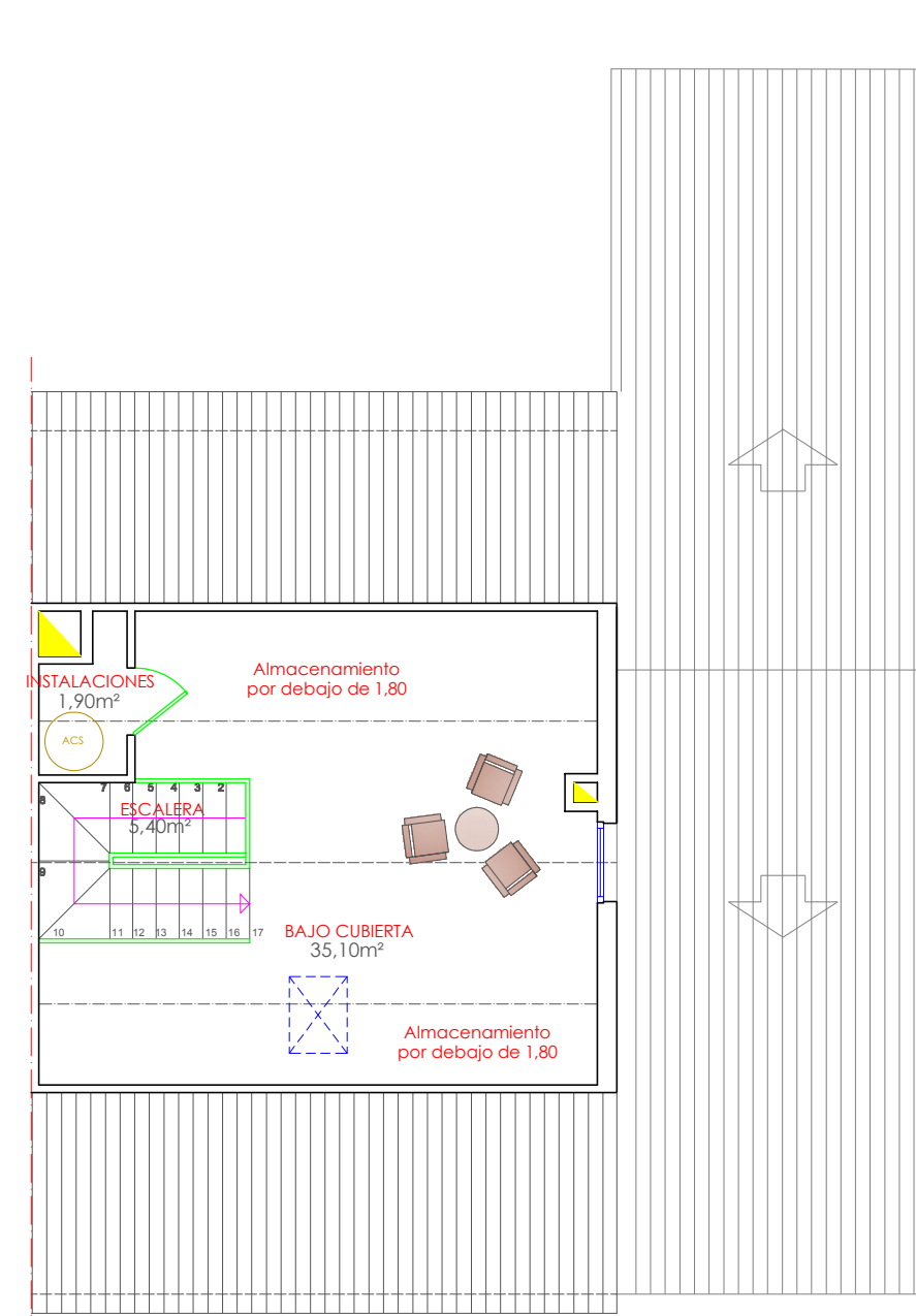
PLANTA BAJOCUBIERTA
