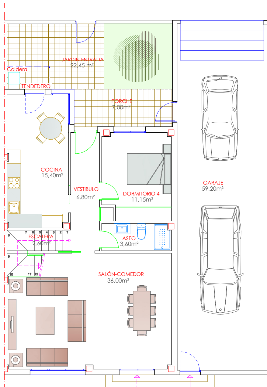
PLANTA BAJA
